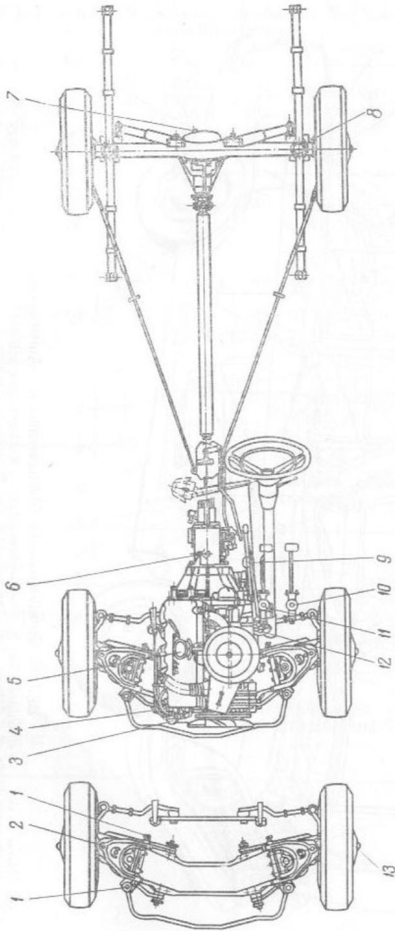
Bild 27. Schmierplan der Fahrgestellmechanismen
