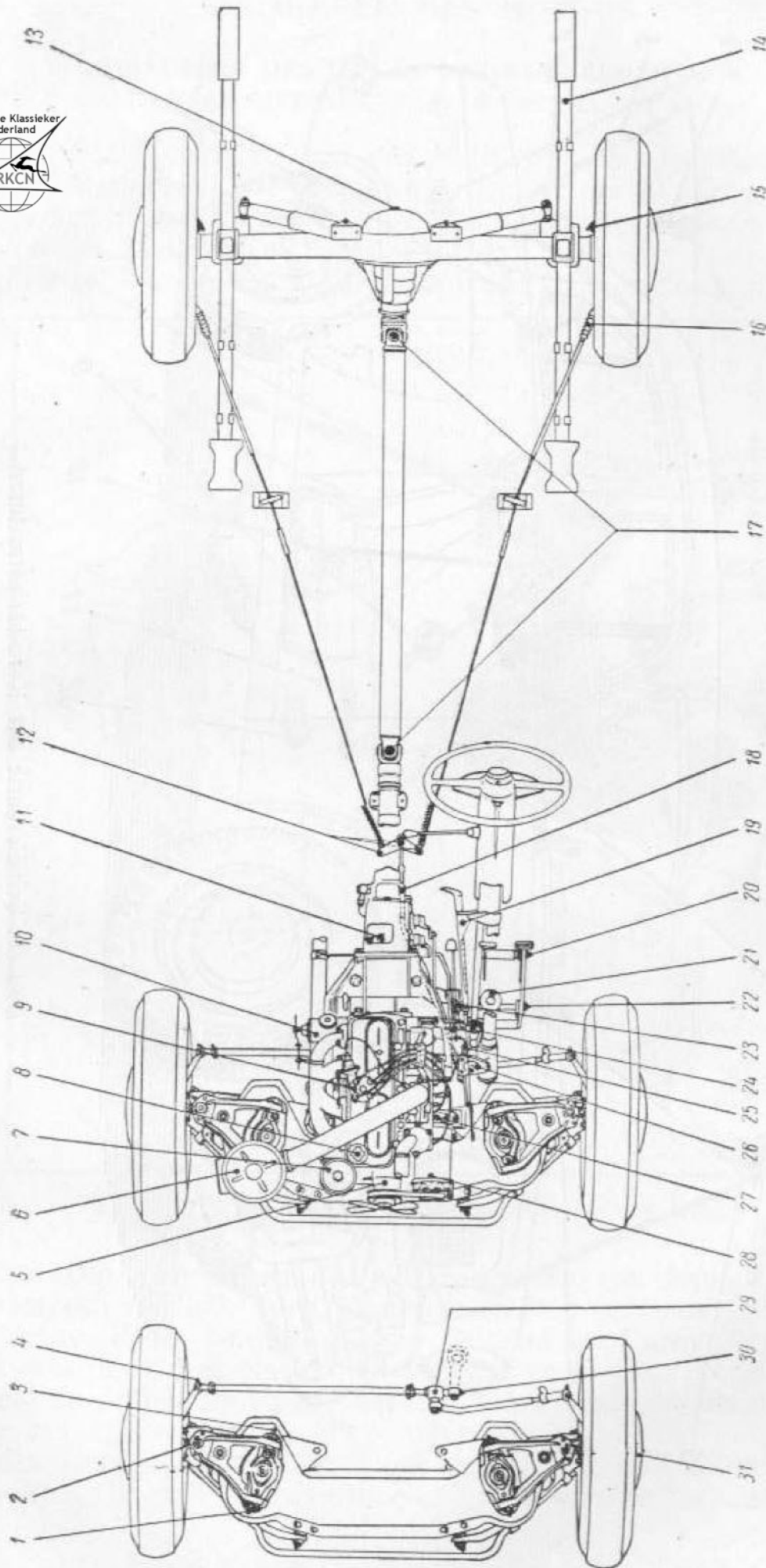
Bild 58. Schmierkarte des Fahrwerks
